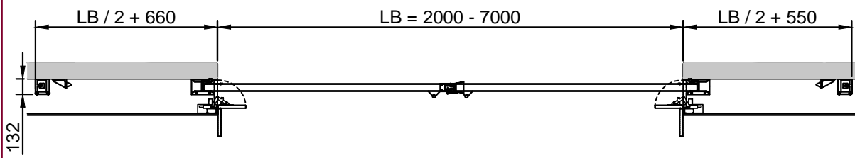
Horizontalschnitt
