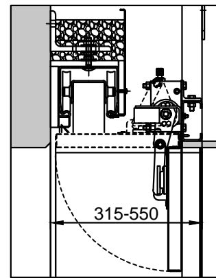
Deckenklappe "optional"
