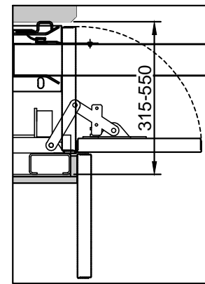
Seitenklappe "optional"
