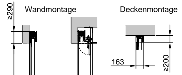
Vertikalschnitt
