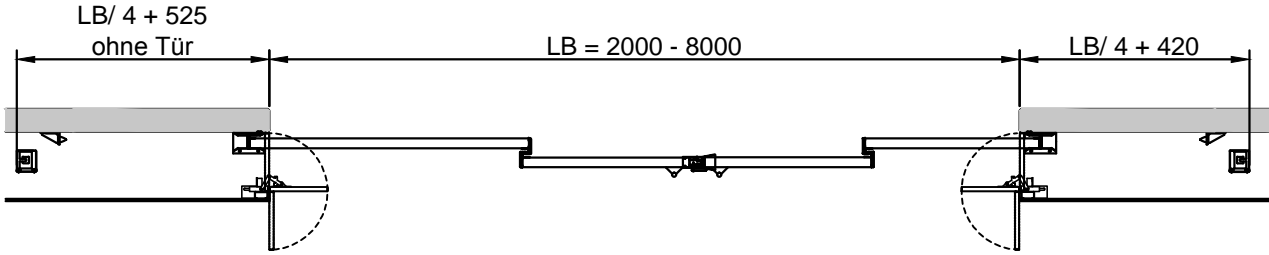
Horizontalschnitt
