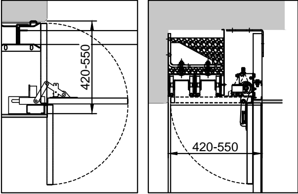
Seitenklappe "optional"
